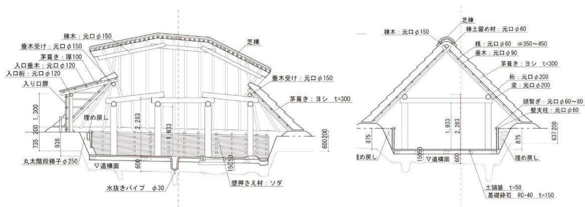
堅穴住居跡復元展示（完全復元）断面図
